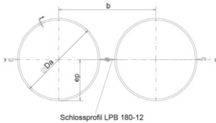
Rohrwand mit LPB 180-12 als Verbinder
